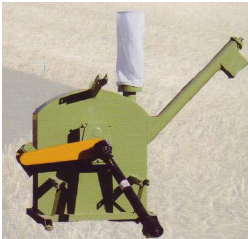
Molino sin mezclador accionado por tractor o electricidad.
